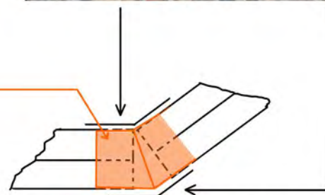
Beispiel einer Eckverbindung aus Zusatzmaterial
